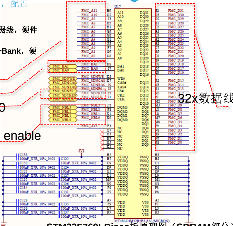
STM32F769I-Disco板原理图（SDRAM部分）
